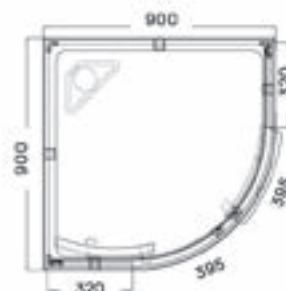
VIVARA HÁTFALAS ZUHANYKABIN TÁLCÁVAL
