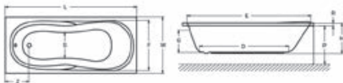
Méreték (mm)
