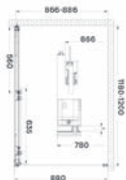
FABIO ZUHANYKABIN
