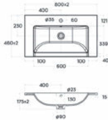
BILBAO 120 MOSDÓSZEKRÉNY
