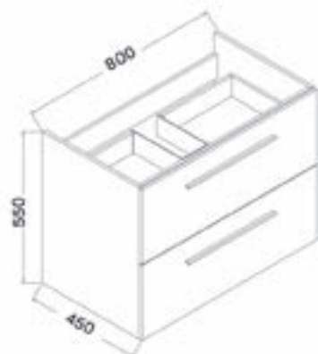
ALMERIA 80 MOSDÓSZEKRÉNY
