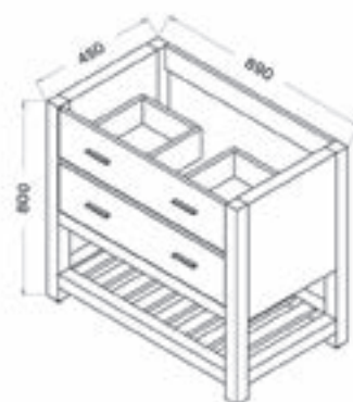
SORIA MOSDÓSZEKRÉNY
