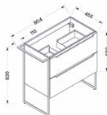
JERSEY MOSDÓSZEKRÉNY
