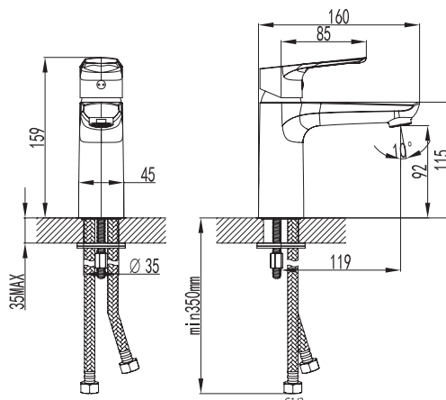
ALTUS MOSDÓ CSAPTELEP
