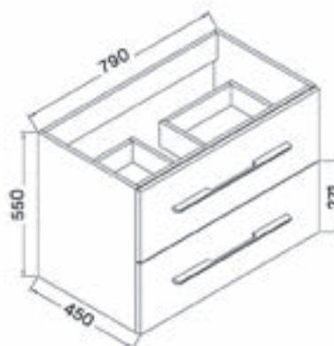
NINA 80 MOSDÓSZEKRÉNY
