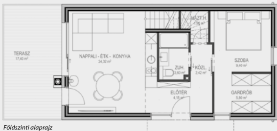
Földszinti alaprajz
