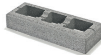
Slim nagykő 60 x 20 x 9 cm
