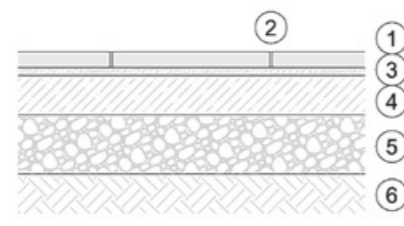
Lapok fektetése habarcságyra (gyalogos forgalmú felületek)
