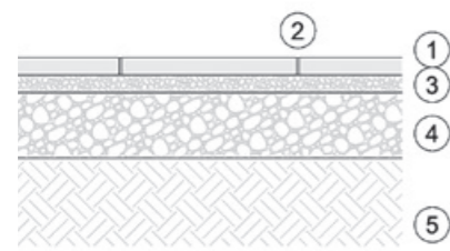
Lapok fektetése kavicságyra (csak gyalogos forgalmú felületek)
