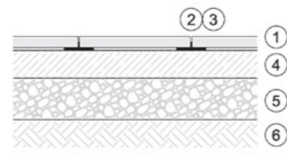
Lapok fektetése laptartó tappancsra (csak gyalogos forgalmú felületek)
